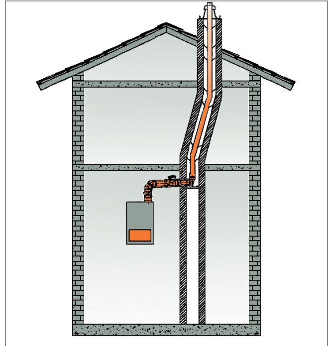
Esempio soluzione di tubo flessibile
