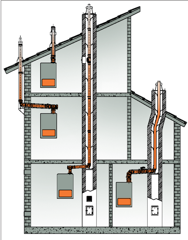
Esempio soluzione di tubo flessibile
