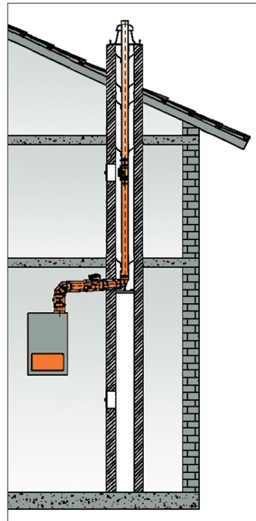
Esempio interno tubo rigido
