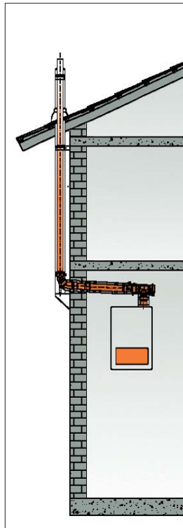
Esempio di una soluzione di LAS esterna
